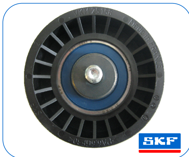
Vezetőgörgő új kialakítás - VKM 25158
